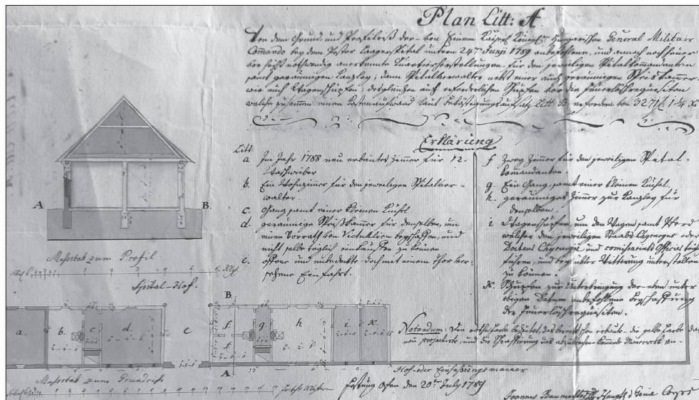
5. kép A pesti Lagerspital tervrajza 82)
