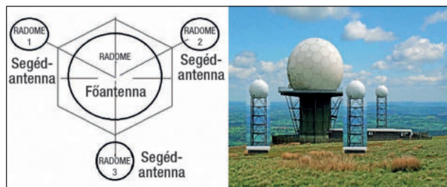
8. ábra. Aktív zavarok és önráveztető rakéták elleni védelem rendszertopológiája (A szerző saját vázlata)
