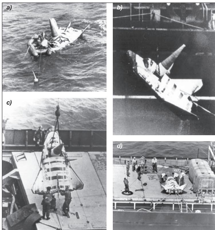
10. ábra. Az ausztrál légierő egyik P-3 Orion típusú felderítő gépe lefényképezte a Kosmosz-1445 néven lajstromozott, visszatért BOR-4 mini-úrrepülőgépet. A fázisképeken a kiemelés látható (Fotók: Royal Australian Air Force)
