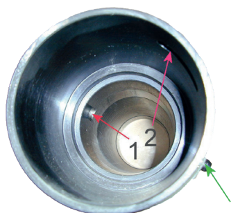
62. ÁBRA. A végére felállított toktest furata szemből nézetben (1. vezetőretest, 2. villaláb- elforduláshatároló hasíték). A zöld nyíl az irányzéktartó mellső illesztő tuskéjének kilátszó végére mutat)
