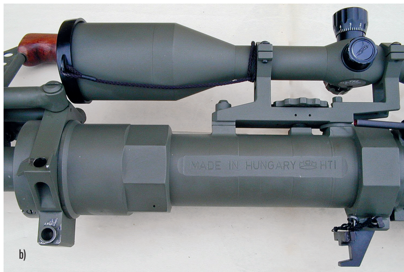
59. ÁBRA. A szerelt tok két változatban. Az a) ábrán három lábon és szerelt csővel, továbbá hátsó lábbal kiegészítve, távcsőszerelék nélkül. A b) ábrán felhajtott villalábakkal, szerelt csővel, szerelt tusával és a hátsó PKM-kapcsoló adapterrel, valamint a távcsőszerelékkal kiegészítve
