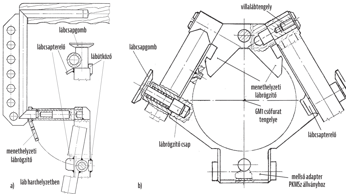
61. ÁBRA. A mellső villalábgyűrű és lábrögzítő szerkezet a) és a hordfogantyú b) szerkezeti ábrája
