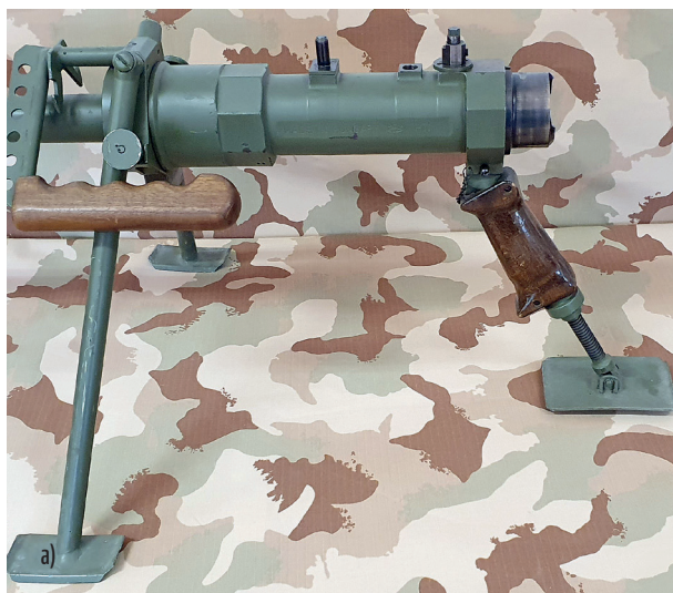
59. ÁBRA. A szerelt tok két változatban. Az a) ábrán három lábon és szerelt csővel, továbbá hátsó lábbal kiegészítve, távcsőszerelék nélkül. A b) ábrán felhajtott villalábakkal, szerelt csővel, szerelt tusával és a hátsó PKM-kapcsoló adapterrel, valamint a távcsőszerelékkal kiegészítve
