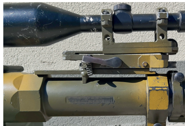
65. ÁBRA. A toktest két nyolcszög keresztmetszetű hasábjának eredeti funkciója. (A kísérleti minta első átalakítása után, a tetejére felszerelt irányzékfelfogó sín lemezének rögzítése, és kitémasztása a toktesthez, továbbá a hátsó adapter/szerelt láb T sín kapcsolatának biztosítása)
