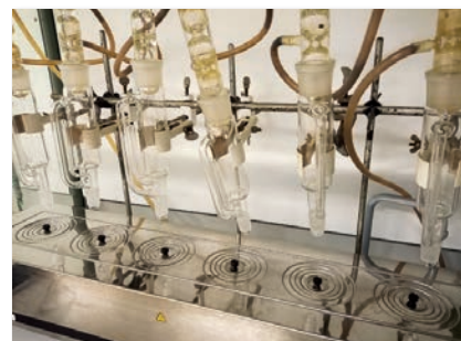
Az üzemanyag-bevizsgáló labor egyik berendezése
